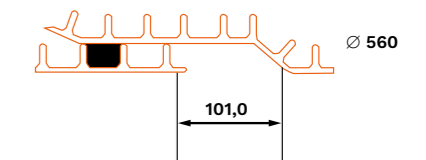
Spoj roztažený 1/10 dy
