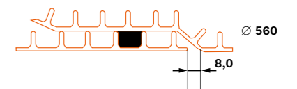
Správné spojení v potrubí Ultra Rib 2
