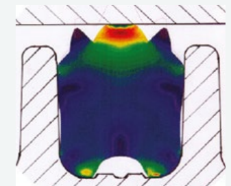
Optimální usazení symetrického těsnění
